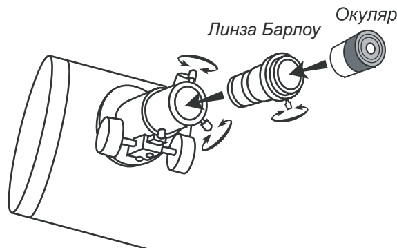
Телескопы-рефлекторы
